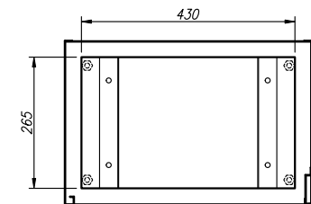
床固定部詳細 (A-A'断面)
