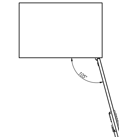
床固定部詳細 (A-A'断面)
