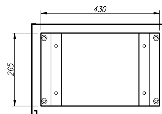
床固定部詳細 (A-A'断面)
